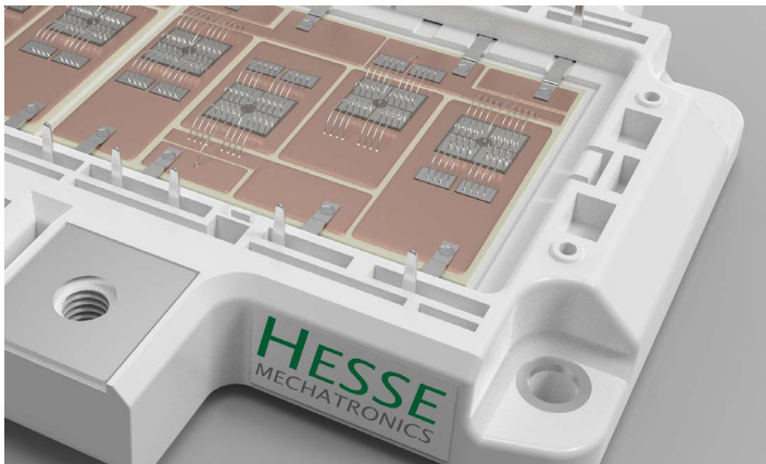
Geschweißtes und gebondetes Power Module
